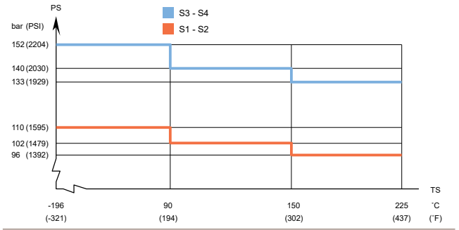
AXP14 - UL 인증 압력/온도 그래프
