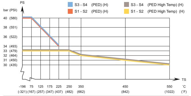
AlfaNova XP27 - PED 인증 압력/온도 그래프
