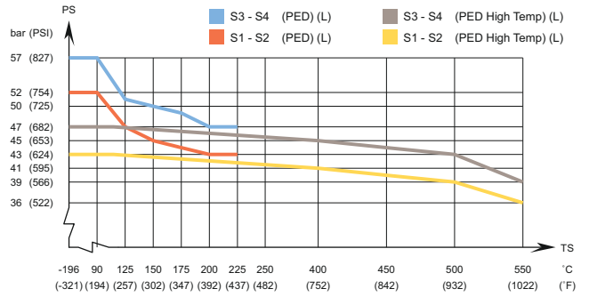
AlfaNova XP27 - PED 고온 인증 압력/온도 그래프
