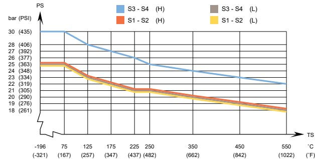
AlfaNova 27 - PED 인증 압력/온도 그래프
