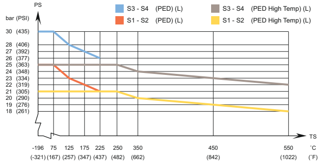
AlfaNova HP 27 - PED 고온 인증 압력/온도 그래프
