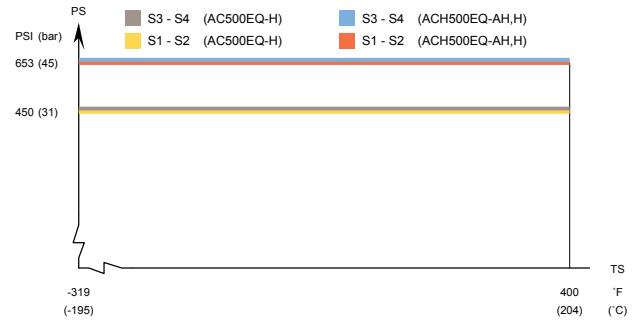
AC500DEQ/ACH500EQ – UL 인증 압력/온도 그래프
