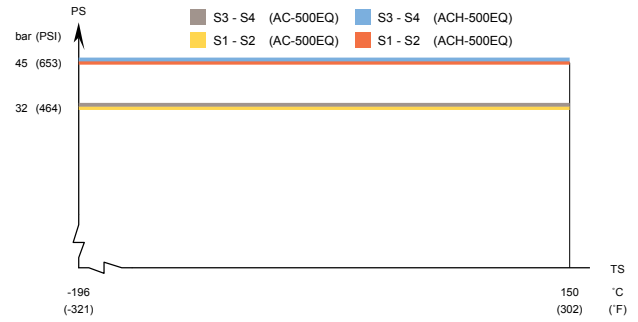
AC500EQ/ACH500EQ – PED 인증 압력/온도 그래프
