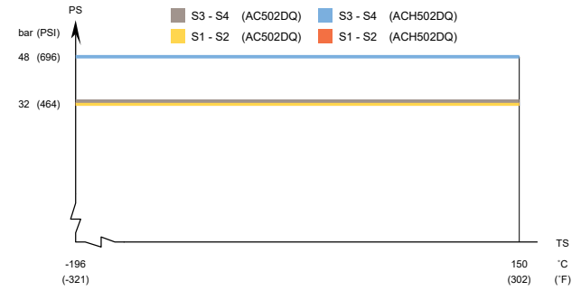
AC502DQ/ACH502DQ – PED 인증 압력/온도 그래프
