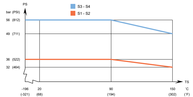
ACK502DQ – PED 인증 압력/온도 그래프
