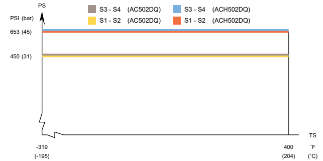
AC502DQ/ACH502DQ – UL 인증 압력/온도 그래프
